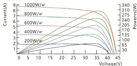
Curva de potência 310W poli I-V a 25°C
