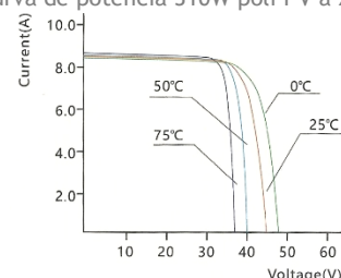
Curva de potência 310W poli I-V a 1000W/m²
